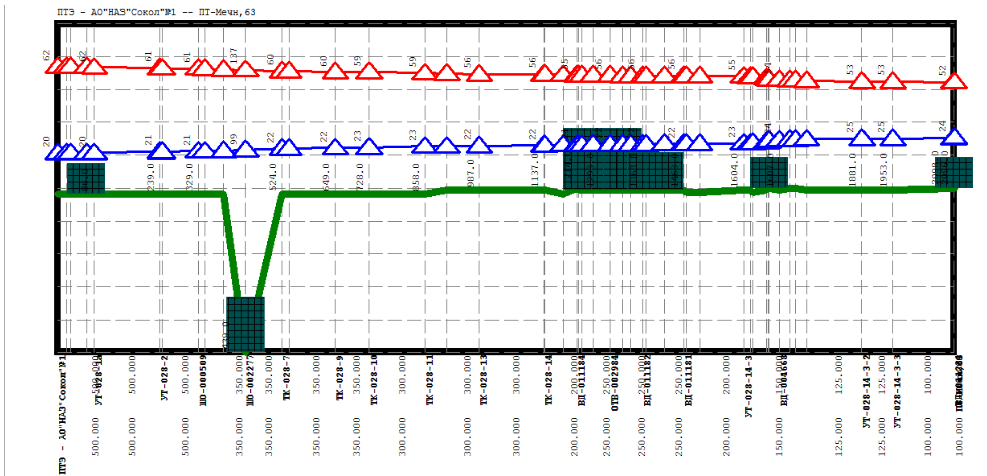
Рисунок 1.94 Результат гидравлического расчета - график гидравлических режимов по пути теплоносителя от котельной Чадаева, 10 до ПТ-Мечн,63
