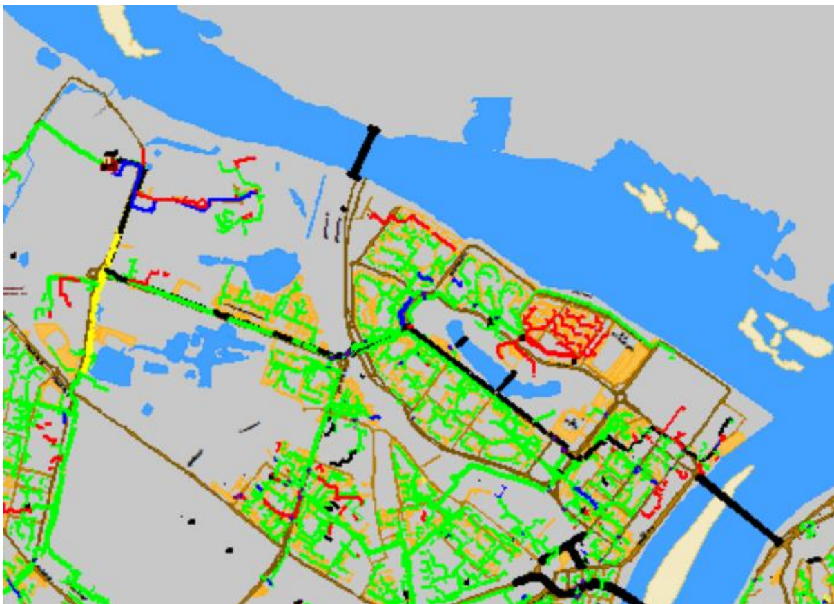
Рисунок 1.5 Результат гидравлического расчета - расчетный путь теплоносителя от СТЭЦ до ПТ-Стрел,19
